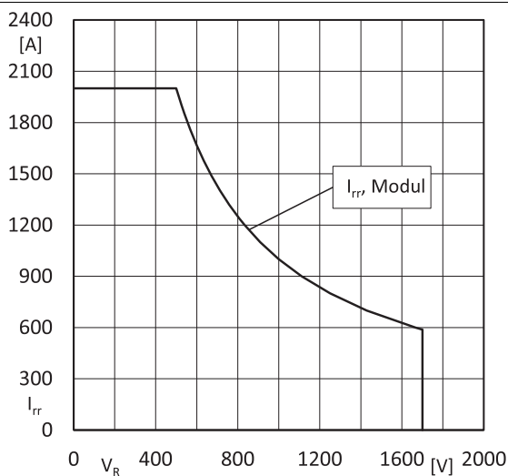
Fig. 11: RBSOA Diode
